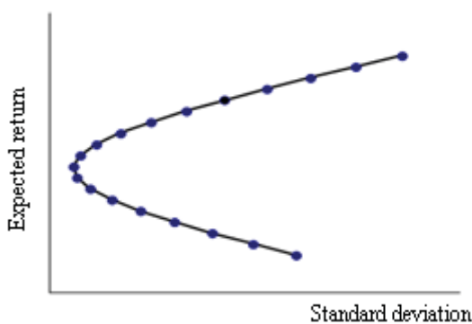
Fig. 1. Efficient frontier
