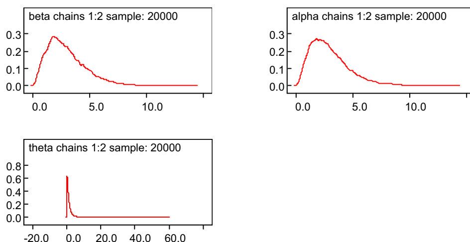
Fig. 1. Posterior densities of parameters of Poisson-Gamma Model
